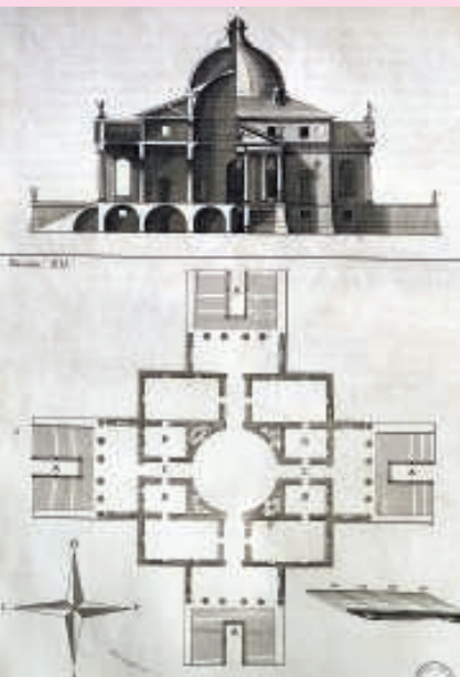
Plattegrond van villa 'La Rotonda'.
